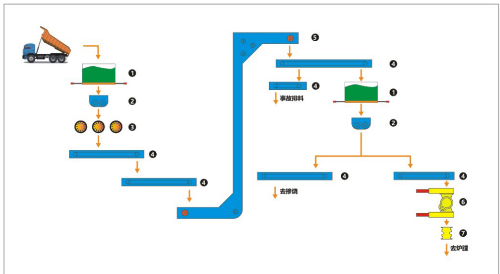
典型干化污泥输送系统工艺图
